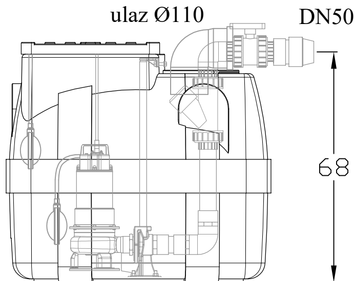
sustav za automatsko spajanje pumpe na tlačni vod s INOX AISI 304 vodilicama i lancem
